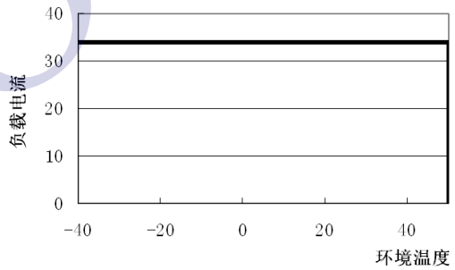
6. 负载电流—环境温度降额曲线 (48V 输出电压):
