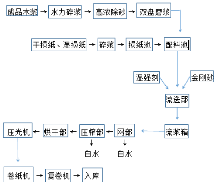
图 2.2-3 2400 纸机生产工艺流程图
