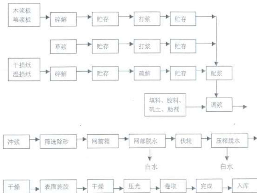
图 2.2-1 抄纸工程生产工艺及流程
