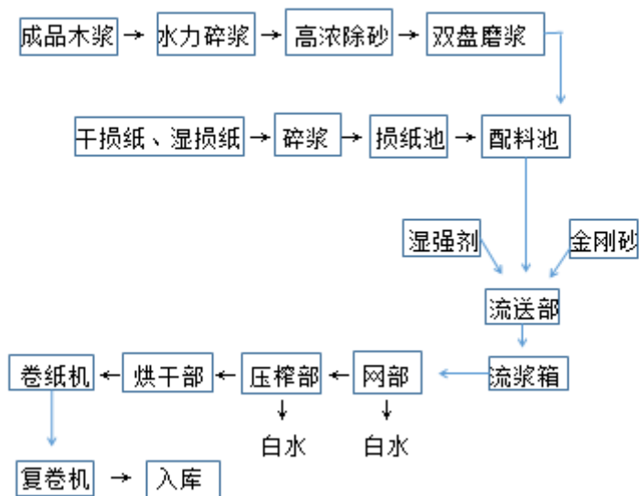
图 2.2-2 1260 纸机生产工艺流程图
