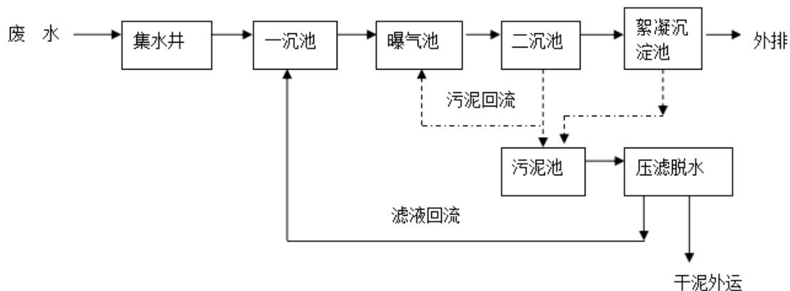
图 2.2-6 4万 m 3 /d 污水处理工艺流程图
